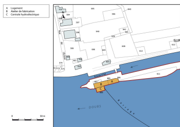
Plan-masse et de situation. Extrait du plan cadastral, 2015, section A. Dess. Mathias Papigny IVR43_20152502656NUDA
