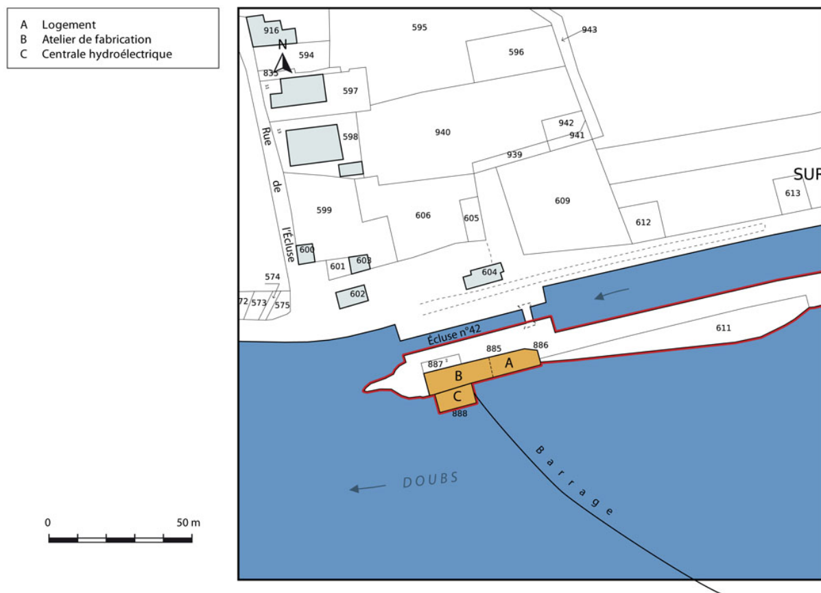
Plan-masse et de situation. Extrait du plan cadastral, 2015, section A.
