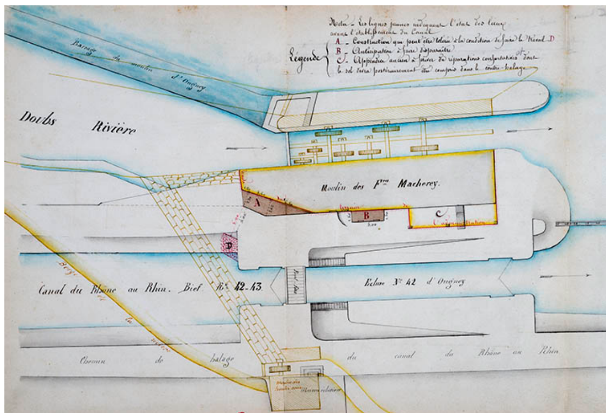
Plan du moulin d'Ougney et de ses abords, 1861.
