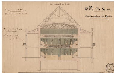
Restauration du théâtre. Coupe transversale sur la salle [projet]. 1844. Phot. Pierre-Marie Barbe-Richaud, Autr. Jacques Athanase Tournour IVR26_20238900281NUC4A
