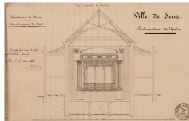
Restauration du théâtre. Coupe transversale sur l'avant-scène [projet]. 1844. Phot. Pierre-Marie Barbe-Richaud, Autr. Jacques Athanase Tournour IVR26_20238900283NUC4A
