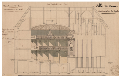
Restauration du théâtre. Coupe longitudinale dans l'axe [projet]. 1844. Phot. Pierre-Marie Barbe-Richaud, Autr. Jacques Athanase Tournour IVR26_20238900282NUC4A
