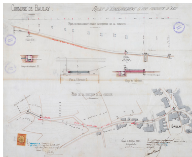
Projet d'établissement d'une conduite d'eau au Nord du village, passant par l'abreuvoir rue de Tallefosse et aboutissant au lavoir, place de la mairie, 1885 Phot. Jérôme Mongreville, Autr. Charles Desgranges IVR43_20167001578NUC4A
