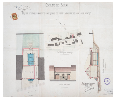
plans du lavoir et remise de matériel à incendie Phot. Jérôme Mongreville, Autr. Charles Desgranges IVR43_20167001566NUC4A
