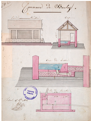
plans du lavoir aujourd'hui disparu Phot. Jérôme Mongreville, Autr. Jean-Baptiste Ridoux IVR43_20167001572NUC4A
