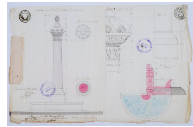
détails fontaine "du haut" Phot. Jérôme Mongreville, Autr. Jean-Baptiste Ridoux IVR43_20167001579NUC4A
