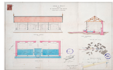
plans du lavoir communal Phot. Jérôme Mongreville, Autr. Charles Humbert IVR43_20167001577NUC4A
