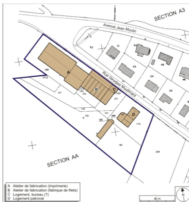
Plan-masse et de situation. Extrait du plan cadastral numérisé, 2008, section AH, 1:1000 réduit à 1:1250. Source : Direction générale des Finances Publiques - Cadastre ; mise à jour : 2008. Dess. André Céréza IVR43_20087000359NUDA
