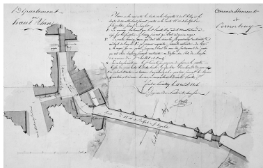
Plan du Grand Pont, 1806. Phot. Yves Sancey, Autr. Stoltz IVR43_19872500072V
