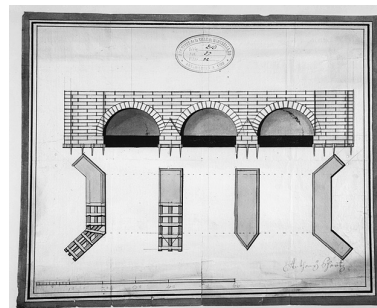
Projet pour la chaussée du Grand Pont, vers 1736. Phot. Jérôme Mongreville, Phot. Anthonus Schrotz IVR43_19872500130V
