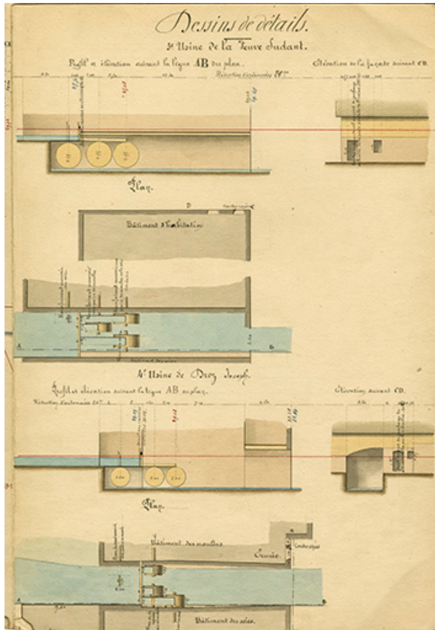
Commune de Grand'Combe. Règlement d'eau des usines [...] Dessins de détails [usines Sudant et Droz], 21 juin 1876.
