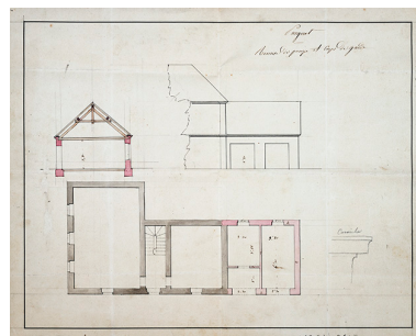
Projet de construction de la remise pour la pompe à incendie, vers 1849. Phot. Jérôme Mongreville, Autr. auteur inconnu IVR43_20187000248NUC4A
