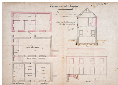
Projet d'aménagement de l'école des filles, 1851. Phot. Jérôme Mongreville, Autr. Adrien Renahy IVR43_20187000247NUC4A
