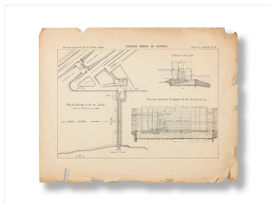
Barrage mobile de Seurre. Plan du barrage et de ses abords. Phot. Thierry Kuntz IVR26_20172100138NUC4A
