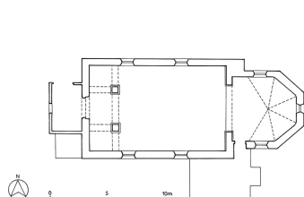
Plan au sol. Phot. Yves Sancey IVR43_19772500298V
