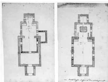
Plan d'agrandissement de l'église, 1846 Phot. Bernard Lardière IVR43_19762500032V
