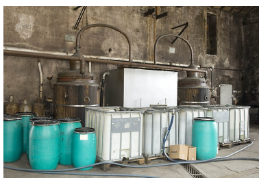
Ancien atelier de distillation. Alambics Egrot-Grangé de 10 hl (mur ouest). Phot. Jérôme Mongreville IVR43_20077000112NUCA
