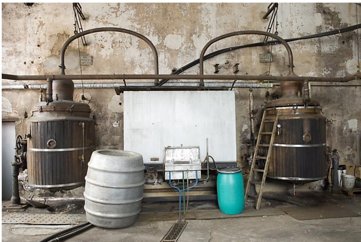
Ancien atelier de distillation. Alambics Egrot-Grangé de 10 hl (mur sud).
