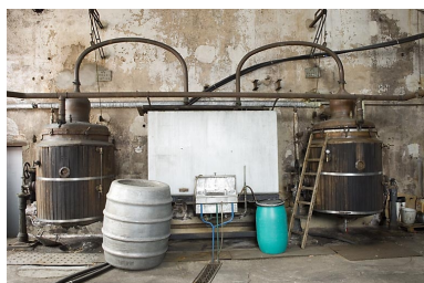
Ancien atelier de distillation. Alambics Egrot-Grangé de 10 hl (mur sud). Phot. Jérôme Mongreville IVR43_20077000111NUCA
