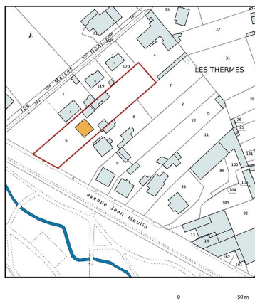
Plan-masse et de situation, extrait du plan cadastral (2021). Dess. Pierre-Marie Barbe-Richaud IVR43_20217000193NUDA
