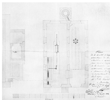
Plan de la localité et dessin géométrique de la chaudière à vapeur pour servir à l'appui de la demande en autorisation adressée à monsieur le préfet du département du Haut-Rhin par M. J. B. Koehl.
