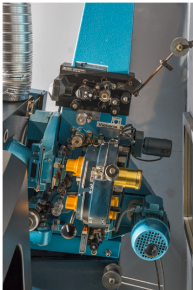
Projecteur argentique 35 mm Cinemeccanica Victoria 5 : Chrono, tourelle porte-objectifs et module son. Phot. Pierre-Marie Barbe-Richaud IVR26_20257100187NUC4A
