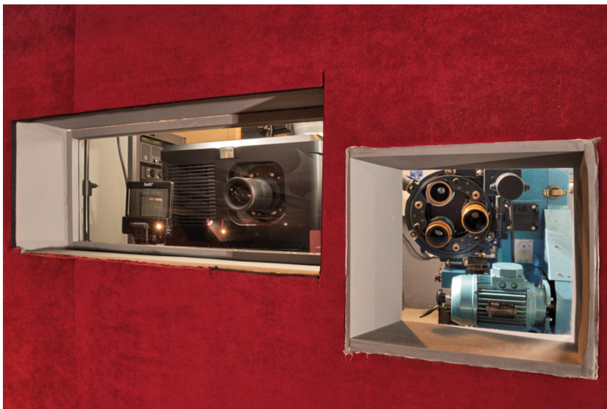
Cabine de la salle 1 (fenêtres depuis la salle) : projecteurs numérique Barco (à gauche) et argentique 35 mm Cinemeccanica Victoria 5.
