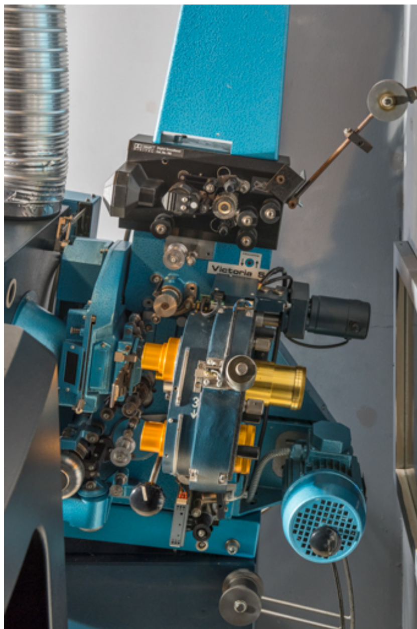
Projecteur argentique 35 mm Cinemeccanica Victoria 5 : Chrono, tourelle porte-objectifs et module son.
