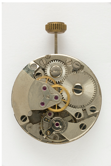
Mouvement Parrenin HP 90 : face côté ponts. Phot. Sonia Dourlot IVR43_20162500734NUC4A
