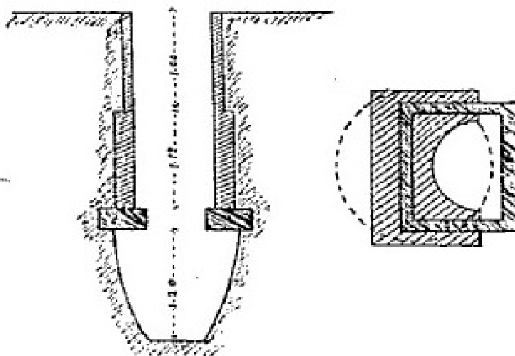
Fig. 63. — COUPE ET PLAN DU CAP- TAGE DE LA SOURCE DE MAIZIÈRES. D'après M. l'ingénieur De Launay.
