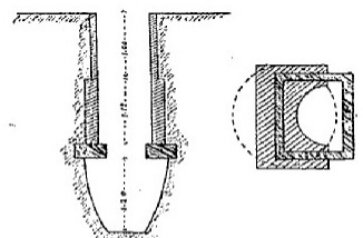
Fig. 63. — COUPE ET PLAN DU CAP- TAGE DE LA SOURCE DE MAIZIÈRES. D'après M. l'ingénieur De Launay.
