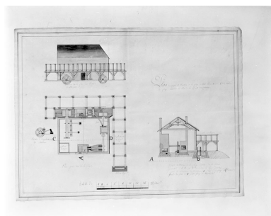
Plan des coupes et élévation de la forge de Mr Pierre Xavier Girod [...].
