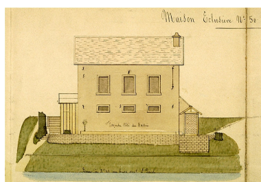
Maison éclusière n° 50 à St Paul - 1880 [détail : ] Façade côté du bassin. Phot. Jérôme Mongreville, Phot. Paul Schoendoerffer IVR43_20012500074XA
