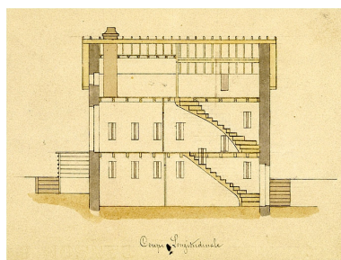
Maison éclusière n° 50 à St Paul - 1880 [détail : ] Coupe longitudinale. Phot. Jérôme Mongreville, Phot. Paul Schoendoerffer IVR43_20012500080XA
