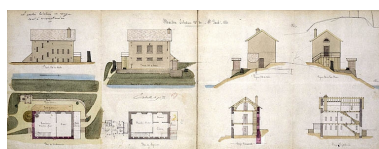
Maison éclusière n° 50 à St Paul - 1880. Phot. Jérôme Mongreville, Phot. Paul Schoendoerffer IVR43_20012500070VA
