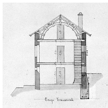
Maison éclusière n° 50 à St Paul - 1880 [détail : ] Coupe transversale. Phot. Jérôme Mongreville, Phot. Paul Schoendoerffer IVR43_20012500081X
