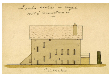
Maison éclusière n° 50 à St Paul - 1880 [détail : ] Façade côté du Doubs. Phot. Jérôme Mongreville, Phot. Paul Schoendoerffer IVR43_20012500072XA
