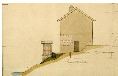
Maison éclusière n° 50 à St Paul - 1880 [détail : ] Pignon côté du moulin. Phot. Jérôme Mongreville, Phot. Paul Schoendoerffer IVR43_20012500076XA
