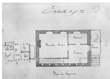
Maison éclusière n° 50 à St Paul - 1880 [détail : ] Plan du logement [au rez-de-chaussée]. Phot. Jérôme Mongreville, Phot. Paul Schoendoerffer IVR43_20012500082X
