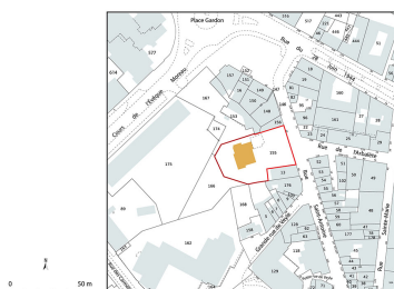
Plan de situation du temple de Mâcon - échelle 1/1000e. Dess. Aline Thomas IVR26_20237100024NUDA
