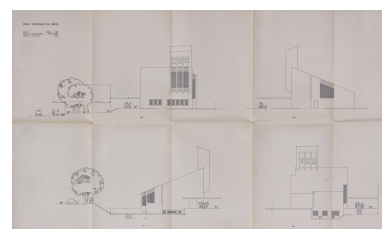
Avant projet de l'église protestante de Mâcon, élévation des quatre façades. Phot. Pierre-Marie Barbe- Richaud, Autr. Oskar Bitterli, Autr. Fernande Bitterli IVR26_20227100252NUC4A
