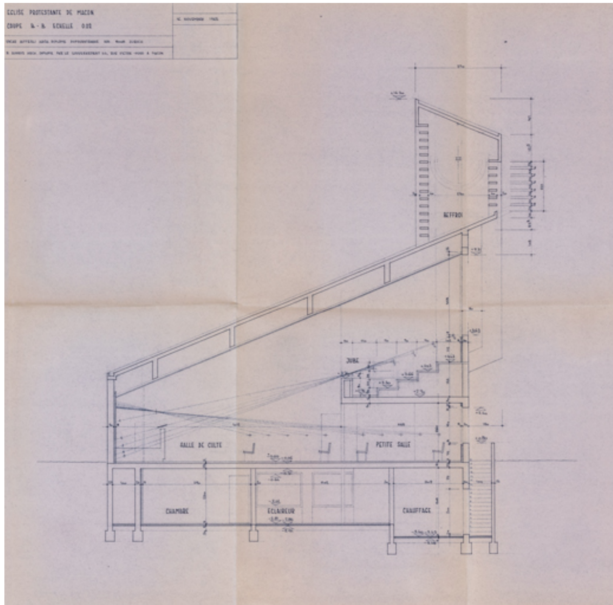
Coupe du temple.
