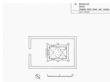
Plan au sol : relevé- croquis G. Poinso, 1975. Phot. Dominique et Sancey Dominguez IVR43_19792500005V
