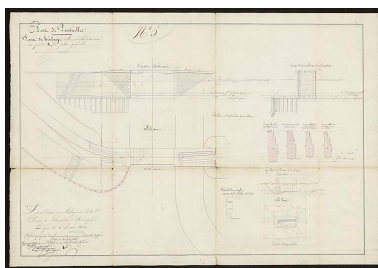
Port de Pontailler. Pont de halage à l'amont de la dérivation au point K du plan général. 1835. Phot. Petot Frédéric IVR26_20202100115NUC4A
