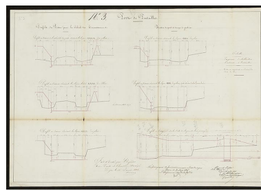
Port de Pontailler. [Profils du port pour le calcul des terrassements]. 1835 Phot. Petot Frédéric IVR26_20202100118NUC4A
