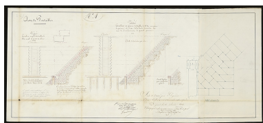
Port de Pontailler. [Escaliers. Coupes et élévations.]. 1835. Phot. Petot Frédéric IVR26_20202100117NUC4A
