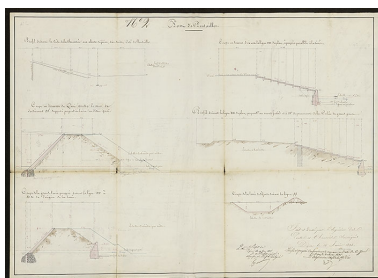
Port de Pontailler. [Coupes et profils]. 1835. Phot. Petot Frédéric IVR26_20202100119NUC4A
