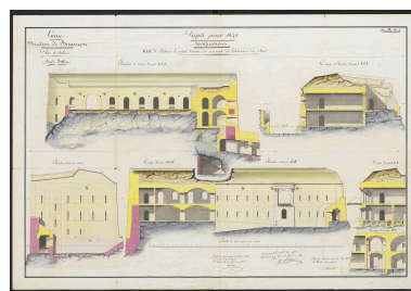
Place de Salins. Fort Belin. Projets pour 1841. Fortifications. Art 3. Achever le réduit terrassé et casematé de l'intérieur du fort (feuille n 4). Autr. Chavelet IVR43_20223901206NUC4A
