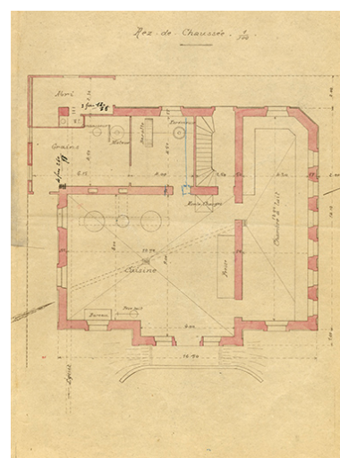
Projet de construction d'un chalet-modèle. Plan du rez-de-chaussée, 1906. IVR43_20192500097NUC4A
