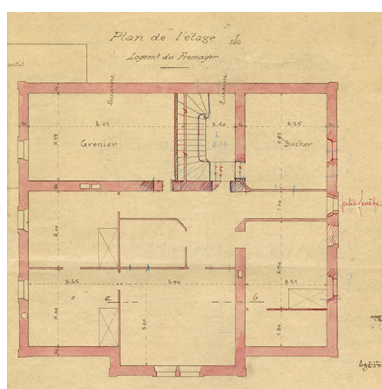
Projet de construction d'un chalet-modèle. Plan de l'étage, 1906. IVR43_20192500095NUC4A
