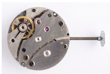
1er mouvement, côté ponts : vue d'ensemble.
