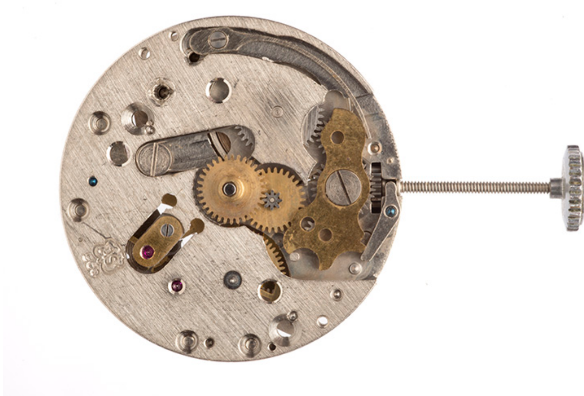
2e mouvement, côté cadran : vue d'ensemble.
