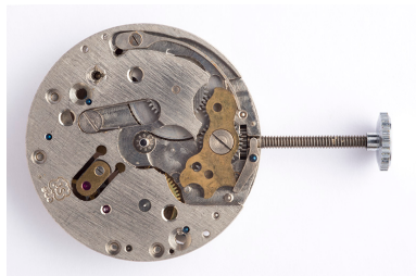
1er mouvement, côté cadran : vue d'ensemble. Il manque au centre la roue de minuterie et sa chaussée.
