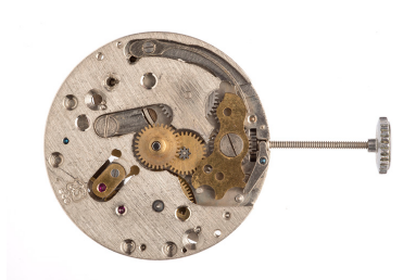
2e mouvement, côté cadran : vue d'ensemble.
