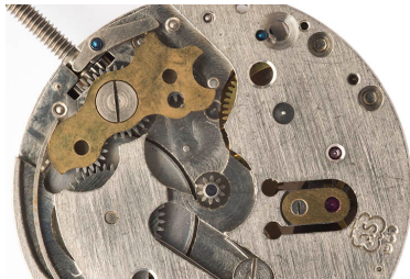
1er mouvement, côté cadran : mécanisme du remontoir. A droite, le logo de la société A. Schild SA.
