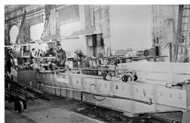
Machine à redresser. Phot. Jérôme Mongreville IVR43_19973901009X
