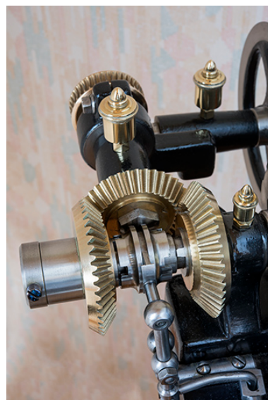
Engrenages et transmission du module de commande. Phot. Sonia Dourlot IVR43_20172500153NUC4A
