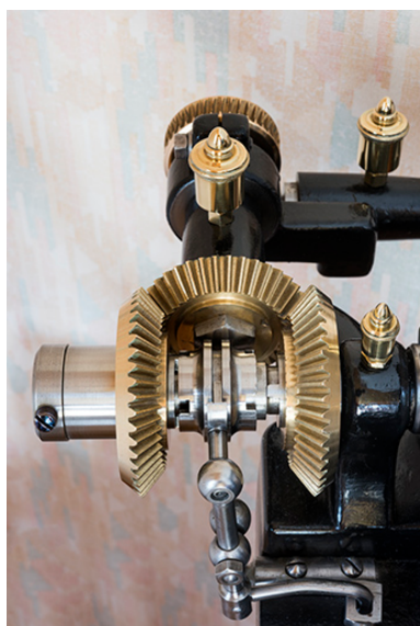
Engrenages et transmission du module de commande.
