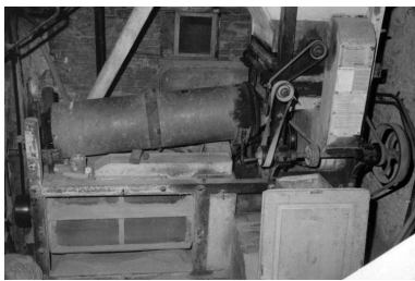
Intérieur : rez-de-chaussée, cage d'escalier, nettoyage combiné. Trémie d'alimentation à droite, cylindre trieur et décortiqueur au centre. Phot. Laurent Poupard IVR43_19883900010Z
