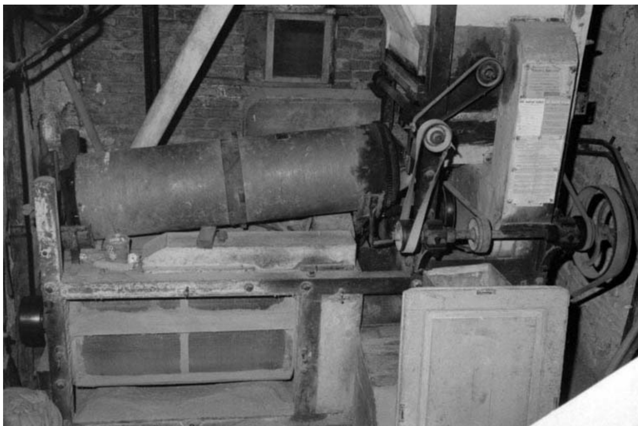
Intérieur : rez-de-chaussée, cage d'escalier, nettoyage combiné. Trémie d'alimentation à droite, cylindre trieur et décortiqueur au centre.
