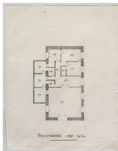
Établissement d'hydrothérapie, plan du rez-de-chaussée, état en 1947. Phot. Pierre-Marie Barbe- Richaud, Autr. auteur inconnu IVR26_20205800003NUC2A
