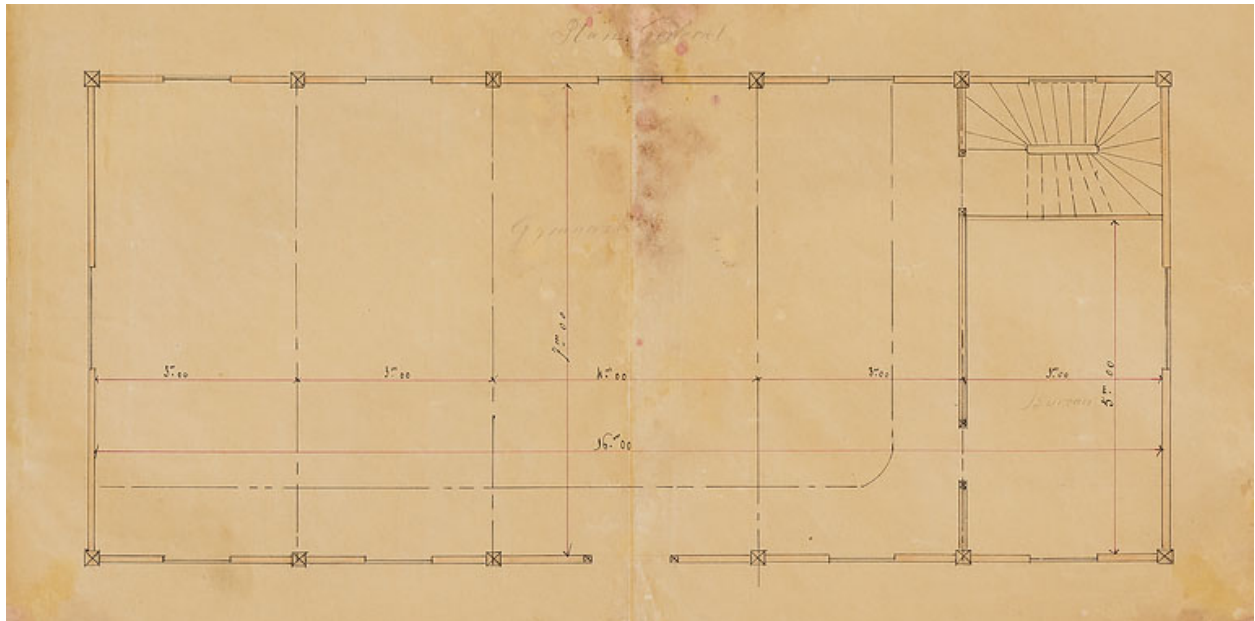
Projet de gymnase, plan.
