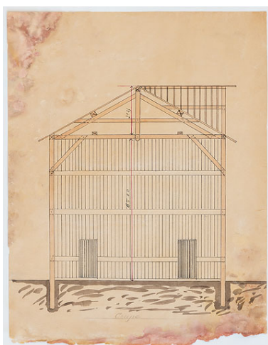
Projet de gymnase, coupe transversale. Repro. Pierre-Marie Barbe- Richaud, Autr. auteur inconnu IVR26_20205800199NUC2A
