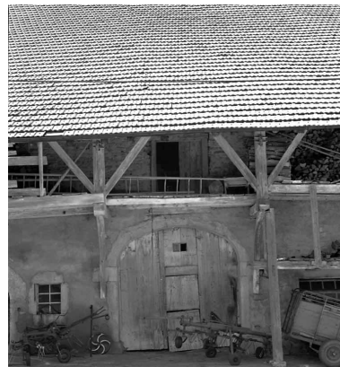
Détail du goutterot sur rue vu de face. Phot. Dominique Dominguez IVR43_19792501010X
