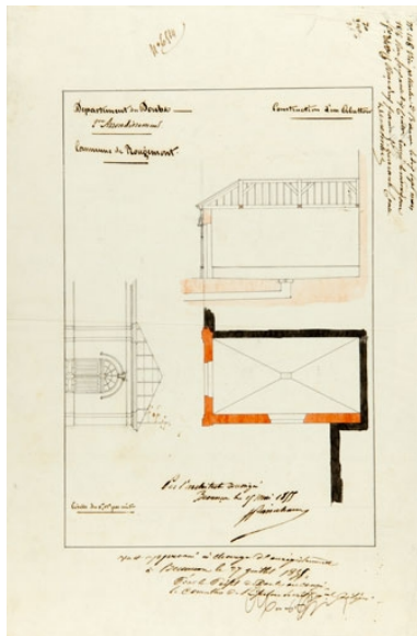
Commune de Rougemont. Création d'un abattoir. 15 mai 1855. Phot. Jérôme Mongreville, Autr. Painchaux IVR43_20102500555NUC4A
