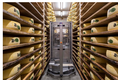
Cave d'affinage : meules de comté et robot de soin JNJ Automation.
