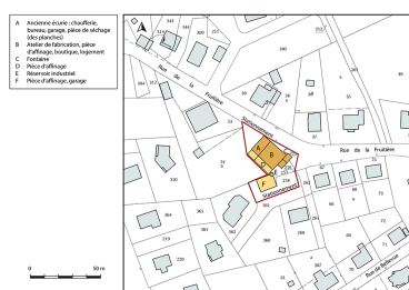
Plan-masse et de situation. Extrait du plan cadastral, 2016, section AE, 1/1 000. Dess. Bertrand Turina IVR43_20182501329NUDA
