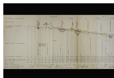
Ligne de Champagnole à Morez. Section de Morbier à Morez. Profil en long du projet dans
