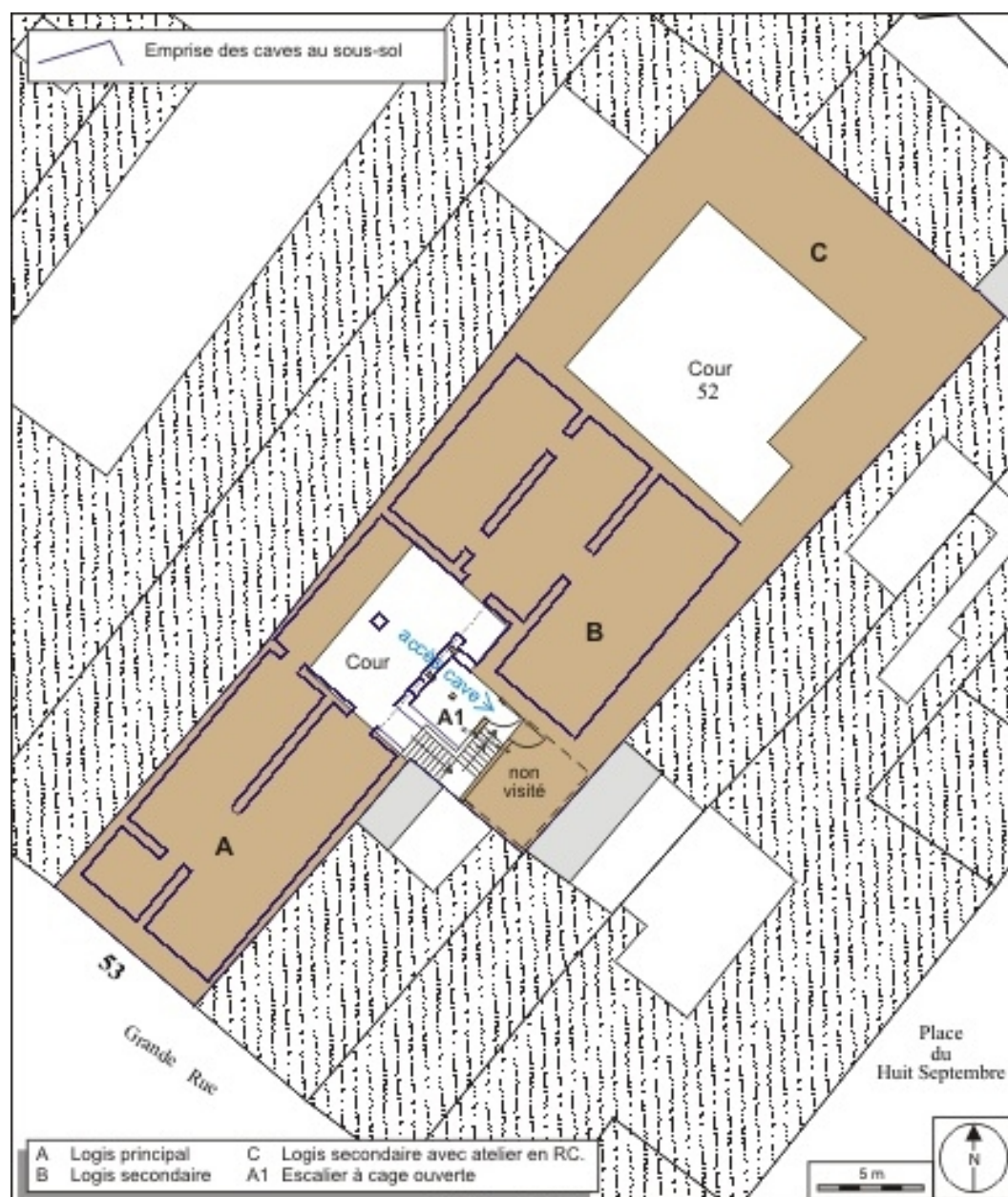
Plan masse du rez-de-chaussée avec implantation des caves. Extrait du plan cadastral, 2007, section AD
