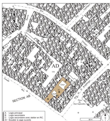
Plan masse et de situation. Extrait du plan cadastral, 1974, section AD. Dess. André Céréza IVR43_20102500062NUDA
