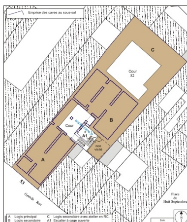
Plan masse du rez-de-chaussée avec implantation des caves. Extrait du plan cadastral, 2007, section AD Dess. André Céréza IVR43_20122500001NUDA
