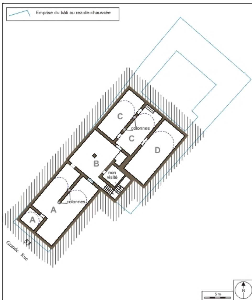
Plan du sous-sol.
