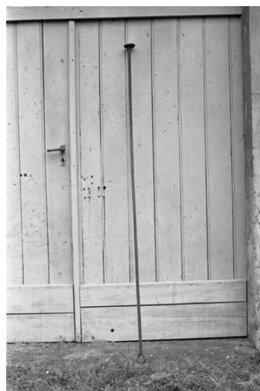
Lance porte-bouchon de fondeur. Phot. Dominique Dominguez IVR43_19817000045Z
