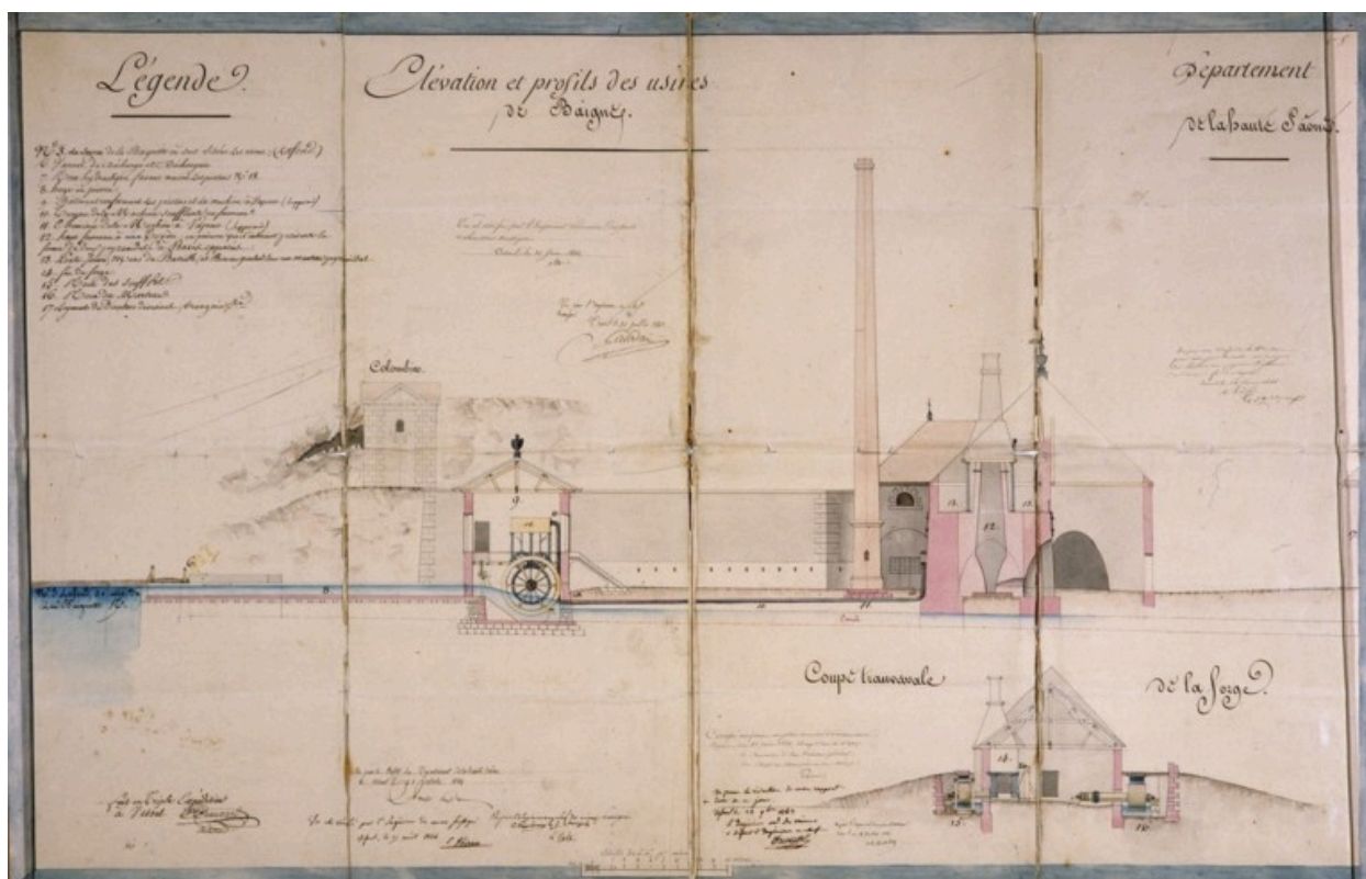
Elévation et profils des usines de Baignes.
