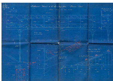
Promenoirs d'Ernest Panz (1895) : détails de l'assemblage des fermes métalliques. Phot. Pierre-Marie Barbe- Richaud, Autr. Ernest Pantz IVR26_20205800247NUC4A
