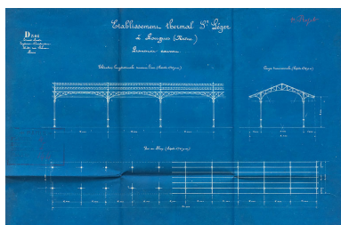
Promenoirs d'Ernest Panz (1895) : plan, coupe et élévation. Phot. Pierre-Marie Barbe- Richaud, Autr. Ernest Pantz IVR26_20205800248NUC4A
