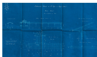
Promenoirs d'Ernest Panz (1895) : plan, coupe et élévation. Phot. Pierre-Marie Barbe- Richaud, Autr. Ernest Pantz IVR26_20205800242NUC2A
