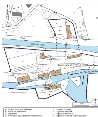
Plan-masse et de situation. Extrait du plan cadastral numérisé, 2008, section AD, 1:1000 réduit à 1:1500. Source : Direction
