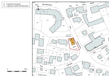
Plan-masse et de situation. Extrait du plan cadastral, 2015, section AI. Dess. Mathias Papigny IVR43_20152502318NUDA
