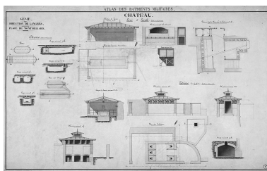
Atlas des bâtiments militaires [...] Feuille 11 [lavoir, lavabo, citernes et latrines], années 1880. Phot. Yves Sancey IVR43_19862500216V
