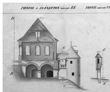
Atlas des bâtiments militaires [... détail de la feuille 5 : élévation de l'ouvrage d'entrée et coupe de l'ancienne chancellerie], 1837. Phot. Jérôme Mongreville, Autr. Le Blanc IVR43_19872500253V
