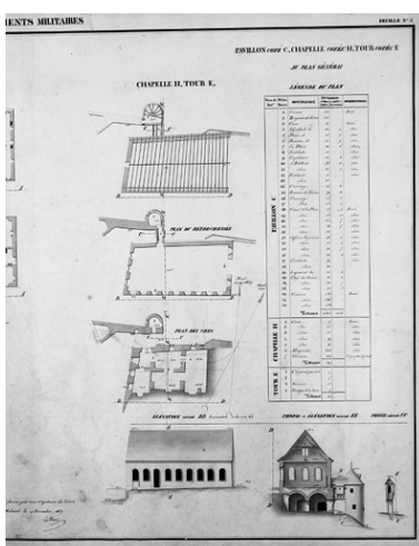
Atlas des bâtiments militaires [... détail de la feuille 5 : ] Chapelle H, Tour E, 1837. Phot. Jérôme Mongreville, Autr. Le Blanc IVR43_19872500252V
