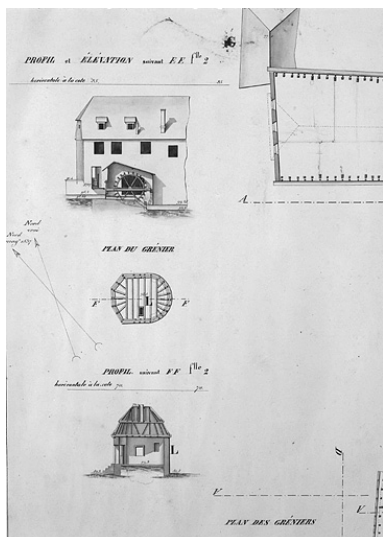
Atlas des bâtiments militaires [...] détail de la feuille 2 : bâtiment de la machine hydraulique et pavillon couronnant la tour L], 1837. Phot. Jérôme Mongreville, Autr. Le Blanc IVR43_19872500258V
