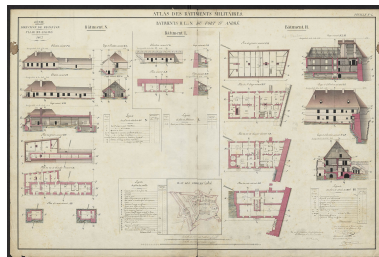
Atlas des bâtiments militaires. Génie. Direction de Besançon. Place de Salins. Bâtiments H, L et N du Fort St-André. 1867. Autr. Jean-Pierre Compas IVR43_20223901217NUC4A
