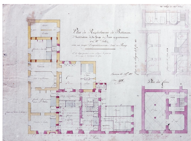
Plan du rez-de-chaussée du bâtiment d'habitation de la forge de Siam appartenant à Mr Jobez avec un projet d'agrandissement tracé en rouge. Phot. Yves Sancey, Phot. Denis-Philibert Lapret IVR43_19923901080XA
