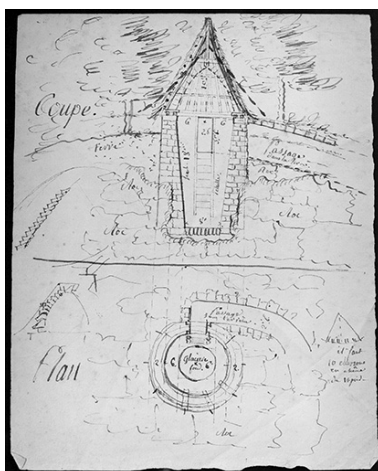
Plan et coupe d'une glacière. Phot. Yves Sancey IVR43_19923901083X
