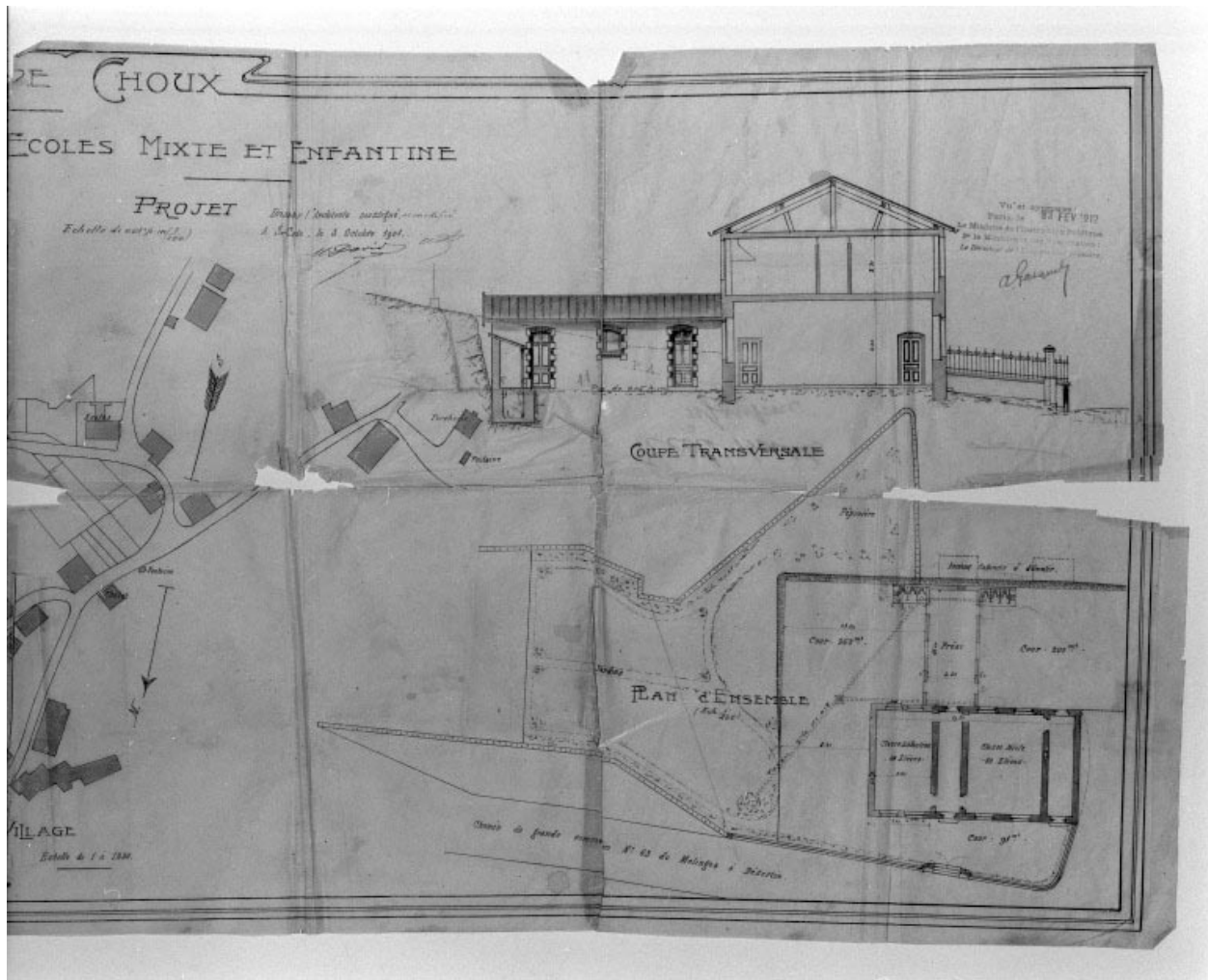
Commune de Choux. Ecoles mixte et infantile. Projet [détail : coupe transversale, plan d'ensemble].
