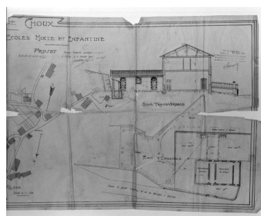
Commune de Choux. Ecoles mixte et enfantine. Projet [détail : coupe transversale, plan d'ensemble]. Phot. Jérôme Mongreville, Autr. Marius (architecte) NEPASUTILISERDavid IVR43_19943901399X
