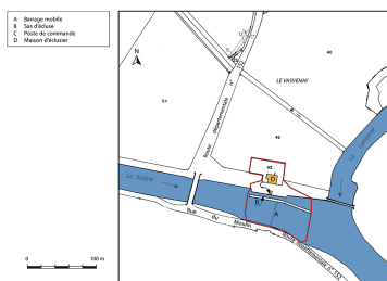
Plan de masse et de situation. Dess. Mathias Papigny IVR43_20177000363NUDA
