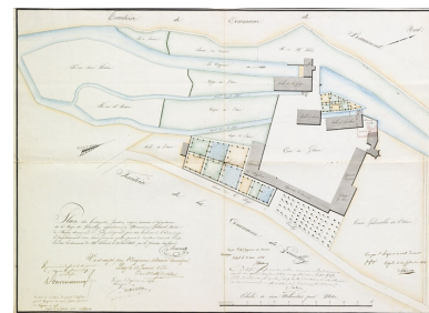
Plan des bâtiments [...], appartenant à monsieur Jobard [...] indiquant par des hachures rouges l'emplacement d'un haut fourneau qu'il se propose de construire [...]. Phot. Jérôme Mongreville, Autr. B. Besancenot IVR43_20097000059NUC2A
