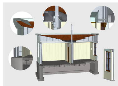
Restitution : coupe de la maison avec détails du système constructif. Dess. Mathias Papigny
