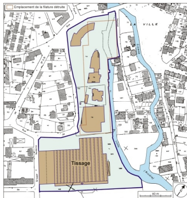
Plan-masse et de situation de l'usine. Extrait du plan
