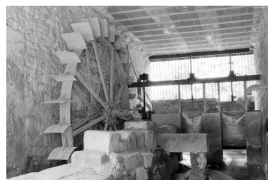
Vannes de prise d'eau, coursiers et roue en dessous. Phot. Laurent Poupard IVR43_19923901218Z
