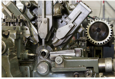
Machine à décolleter Tornos : espace d'usinage (vue rapprochée). Phot. Sonia Dourlot IVR43_20142500714NUC2A
