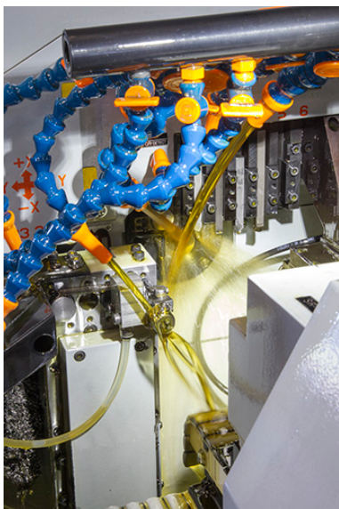
Machine à décolleter Star SR-10J type C : espace d'usinage. Phot. Sonia Dourlot IVR43_20142500710NUC2A
