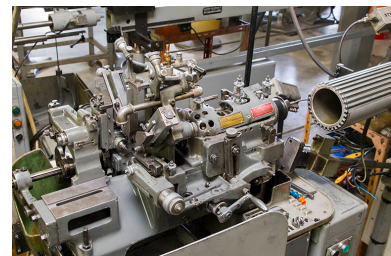
Machine à décolleter Tornos : espace d'usinage. Phot. Sonia Dourlot IVR43_20142500712NUC2A
