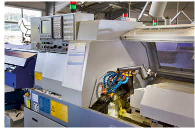
Machine à décolleter Star SR-10J type C : commande et espace d'usinage. Phot. Sonia Dourlot IVR43_20142500709NUC2A
