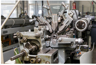
Machine à décolleter Tornos : espace d'usinage et extrémité du ravitailleur. Phot. Sonia Dourlot IVR43_20142500713NUC2A
