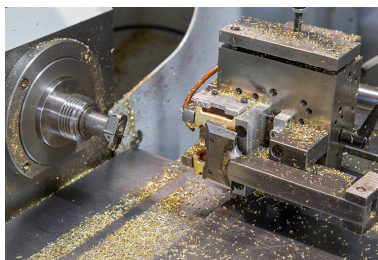
Tour à diamanter (vue rapprochée). Phot. Sonia Dourlot IVR43_20142500705NUC2A
