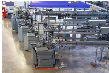
Machines à décolleter Tornos et leurs ravitailleurs (côté sud). Phot. Sonia Dourlot IVR43_20142500700NUC2A
