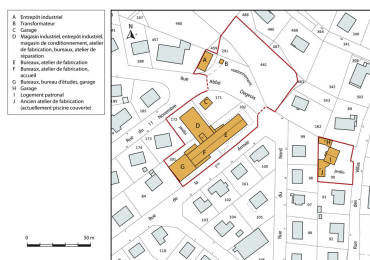
Plan-masse et de situation. Extrait du plan cadastral, 2015, section AB. Dess. Mathias Papigny IVR43_20152500609NUDA
