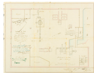
Plan de détail de l'usine à fer du Gouffre du Lod, appartenant à Monsieur A. de Blondeau, maître de forges à St Hippolite, 14 septembre 1852. Phot. Sonia Dourlot IVR43_20192500853NUC4A
