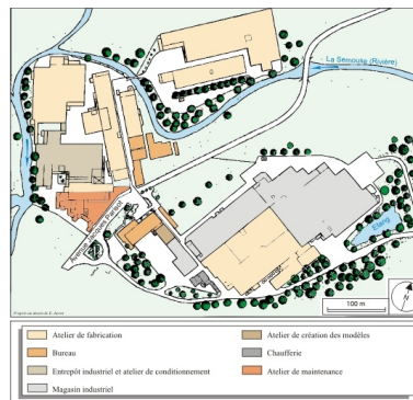
Plan-masse de l'usine. D'après un plan de l'entreprise, mis au net par André Céréza. Dess. André Céréza IVR43_20067000994NUDA
