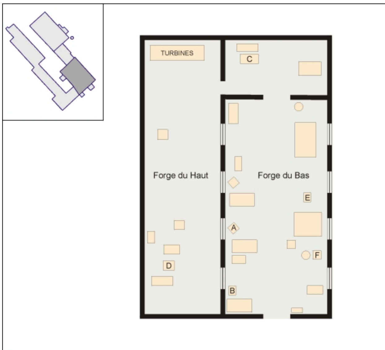
Plan de localisation des fours à gaz.
